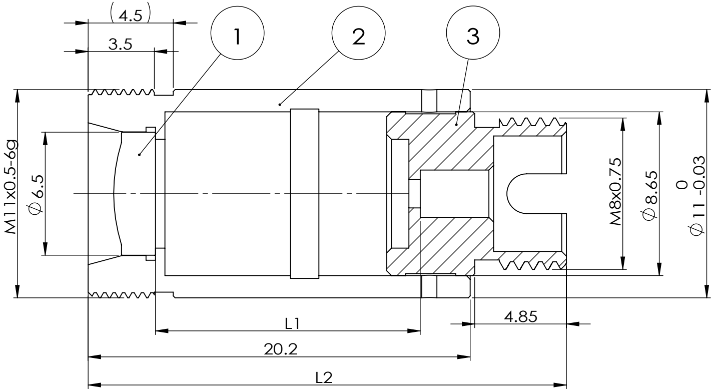
SECTION A-A
